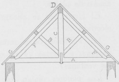
Las partes de una armadura de tejado: A, tirantes; B, jabalcones; C, pendolón; D, hileras; F, pares, y G, parecillos
