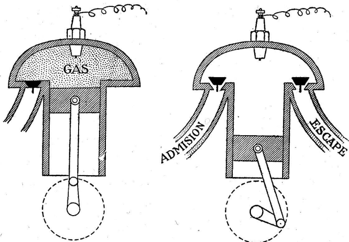
Esquema núm. 6. — El pistón ha comprimido el gas que llena el hueco de la cámara de explosión
