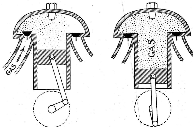
Esquema núm. 8. — El cilindro aspira el gas. La válvula de admisión está abierta y la de escape cerrada (Admisión)
