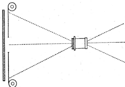
Fig. 18. — El obturador de «plano focal» se compone de una cortinilla que se desliza muy cerca de la placa. Esta cortinilla tiene una abertura variable en el centro, que es por donde los rayos luminosos impresionan la placa
