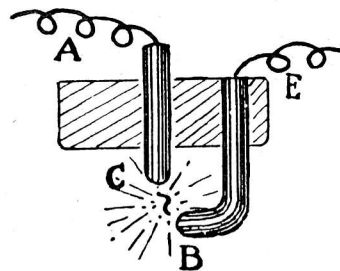
Esquema núm. 15.— Elementos de una «bujía» eléctrica: entrada y salida de la corriente, y puntos donde salta el chispazo
