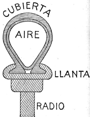
Esquema núm. 52. — Corte transversal de un neumático montado en su llanta
