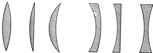
Fig. 4. — Esquema del corte de algunas formas de lentes que se emplean para fabricar objetivos fotográficos. Los tres primeros son convergentes, y los tres últimos divergentes
