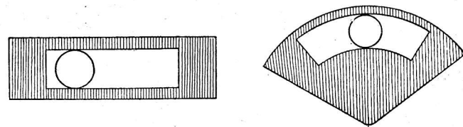
Fig. 17. -- Esquema del obturador llamado «de guillotina». Una placa cuya abertura rectangular se desliza rápidamente entre los lentes, abriendo y cerrando el objetivo o un segmento de círculo que, al girar, hace el mismo efecto
