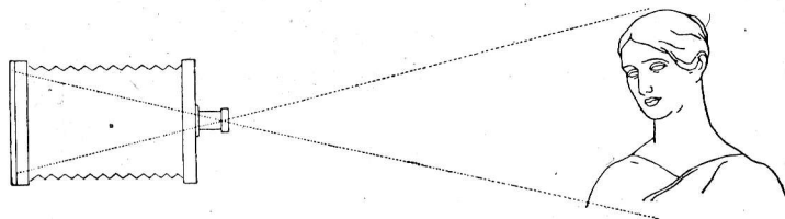
Fig. 13. — Los objetivos para retratos en sus cualidades son lo contrario de un «gran angular», es decir, que se destinan a fotografiar objetos de tamaño reducido (figura humana, cabezas, bustos), un poco alejados de la cámara para evitar deformaciones, y sin que el objeto se reduzca mucho. Tienen «poco ángulo» y son «largos de foco»
