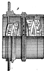
Fig. 10. — Doble anastigmático.
