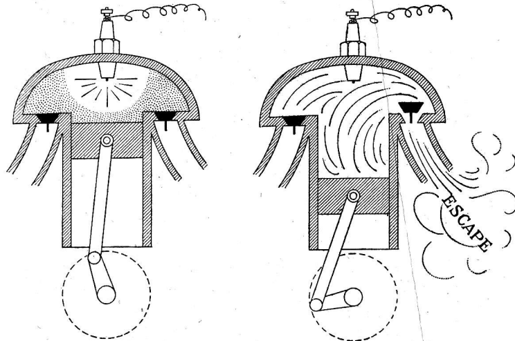
Esquema núm. 10. — El pistón ha comprimido el gas que estalla al saltar el chispazo de la bujía. Ambas válvulas están cerradas (Explosión)
