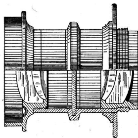
Fig. 7. — Objetivo rectilíneo
