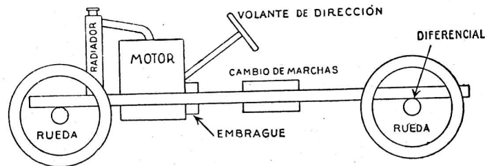
Esquema núm. 47. — Un «chasis» visto de perfil, indicando la situación de los mecanismos. Cada fabricante de automóviles tiene su modelo dotado de características especiales, pero en resumen todos los automóviles se componen de las piezas indicadas en este gráfico y el anterior
