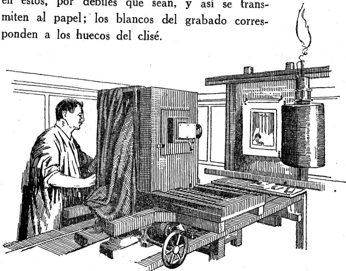
Las máquinas fotográficas que se utilizan para reproducciones destinadas a clisés tipográficos, afectan formas y dispositivos especiales. En el dibujo se representa una cámara con objetivo prismático puesto a un lado; así el negativo no sale invertido, como ocurre en las cámaras ordinarias
