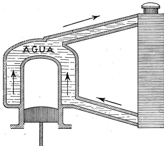
Esquema núm. 19. — El grabado muestra el cilindro rodeado de una doble cubierta llena de agua. Un tubo va a parar a la parte baja del radiador, y otro al extremo superior. Al calentarse el agua se dilata y sube por sí sola, mientras la enfriada desciende. Este sistema es el llamado de «termosifón». En muchos motores la circulación del agua se efectúa por medio de una bomba
