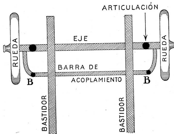
Esquema núm. 37. — El mecanismo para mover las ruedas de un automóvil
