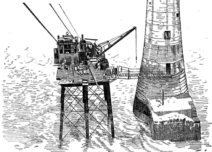
Construcción de un faro dentro del mar, asentando la fábrica en una roca. Desde un acantilado de la costa, por medio de cables, se trasladan los obreros y el material
