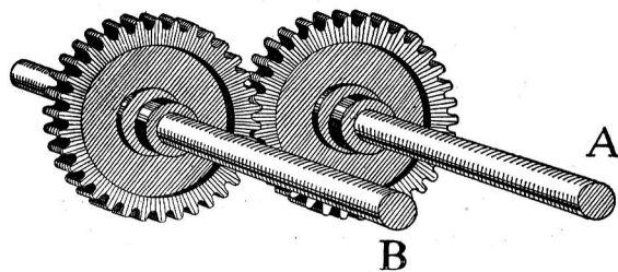
Esquema núm. 29. — Dos ruedas dentadas iguales
