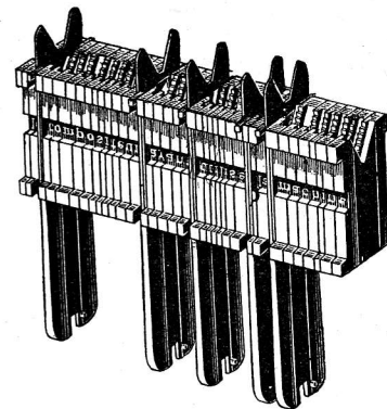
Matrices de una máquina de componer dispuestas para fundir una línea entera. Entre las palabras se muestran los espacios formando cuna. Según estas cuñas se aprietan más se ensancha la línea hasta llegar a la dimensión requerida
